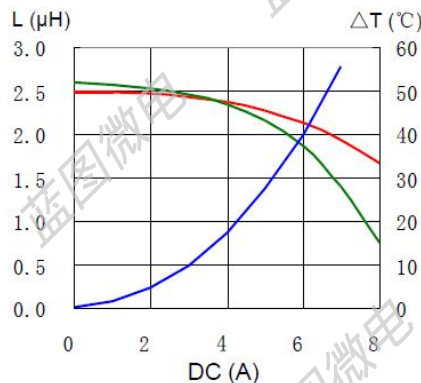
SRH8D38-6R0N
