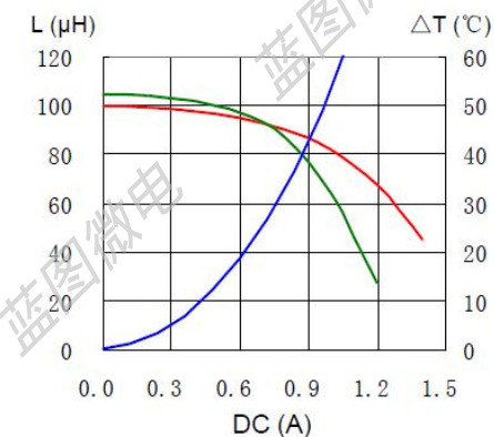
SRH8D38-101N
