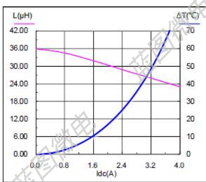
SMS0650-330M
