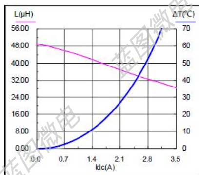
SMS0650-470M
