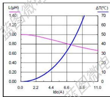
SMS0520-1R0M
